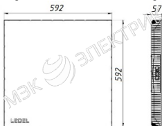
Рисунок 1 Светильник «L-office 32 S Premium/Em»
