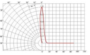
Исполнение «K15»
