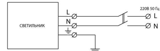
Рисунок 3 Схема подключения светильника
