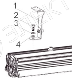
Рисунок 4 Монтаж крепления
