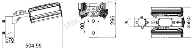
Рисунок 1б Габаритные размеры светильника «L-street 40 Turbine»
