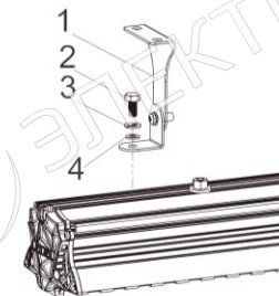
Рисунок 4 Монтаж крепления
